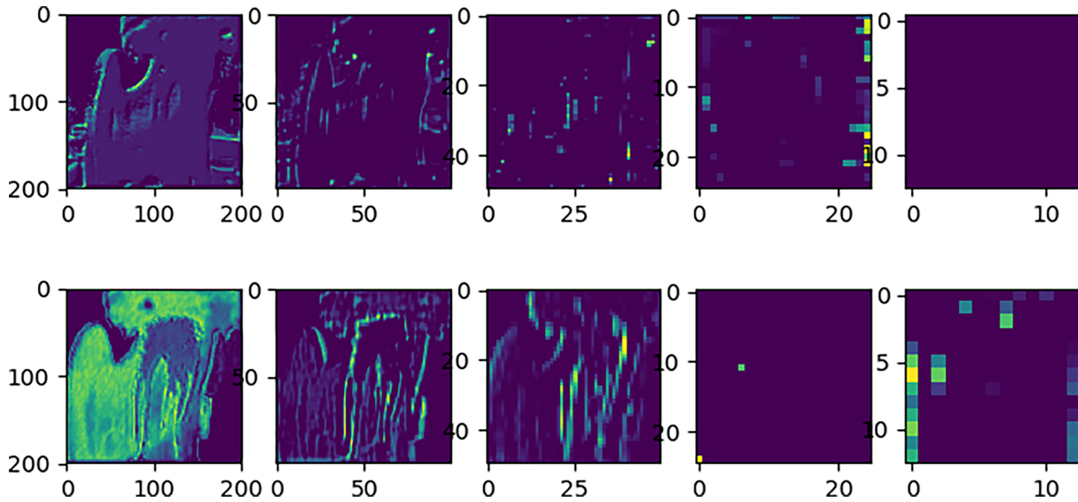
Fig. 4 Feature map.
